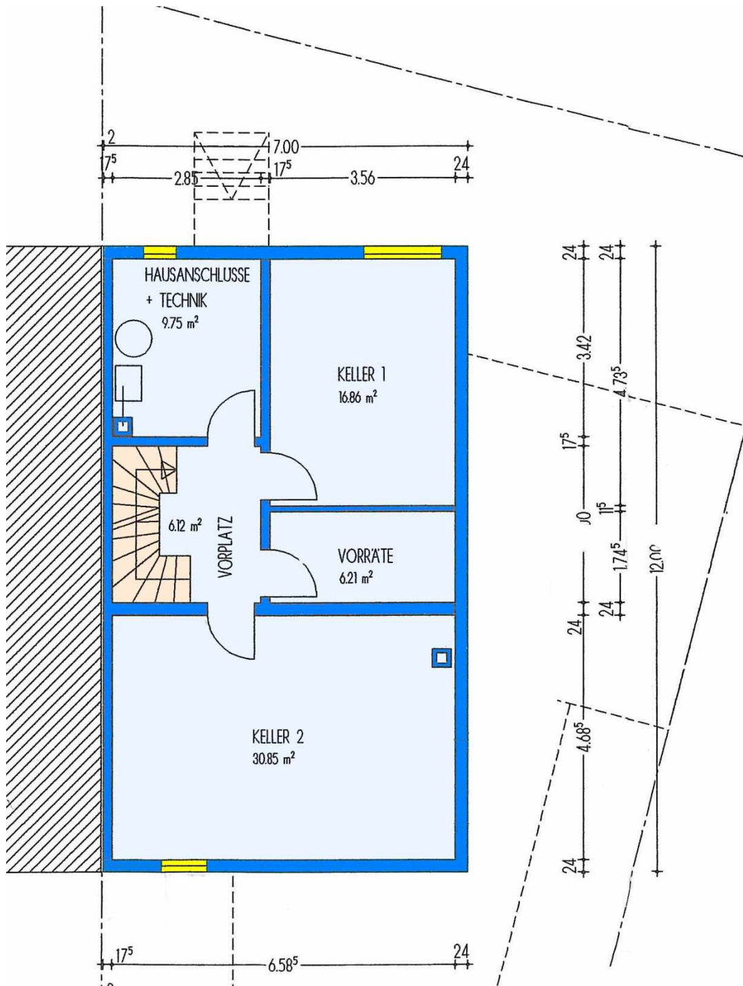
Grundriss Untergeschoss
