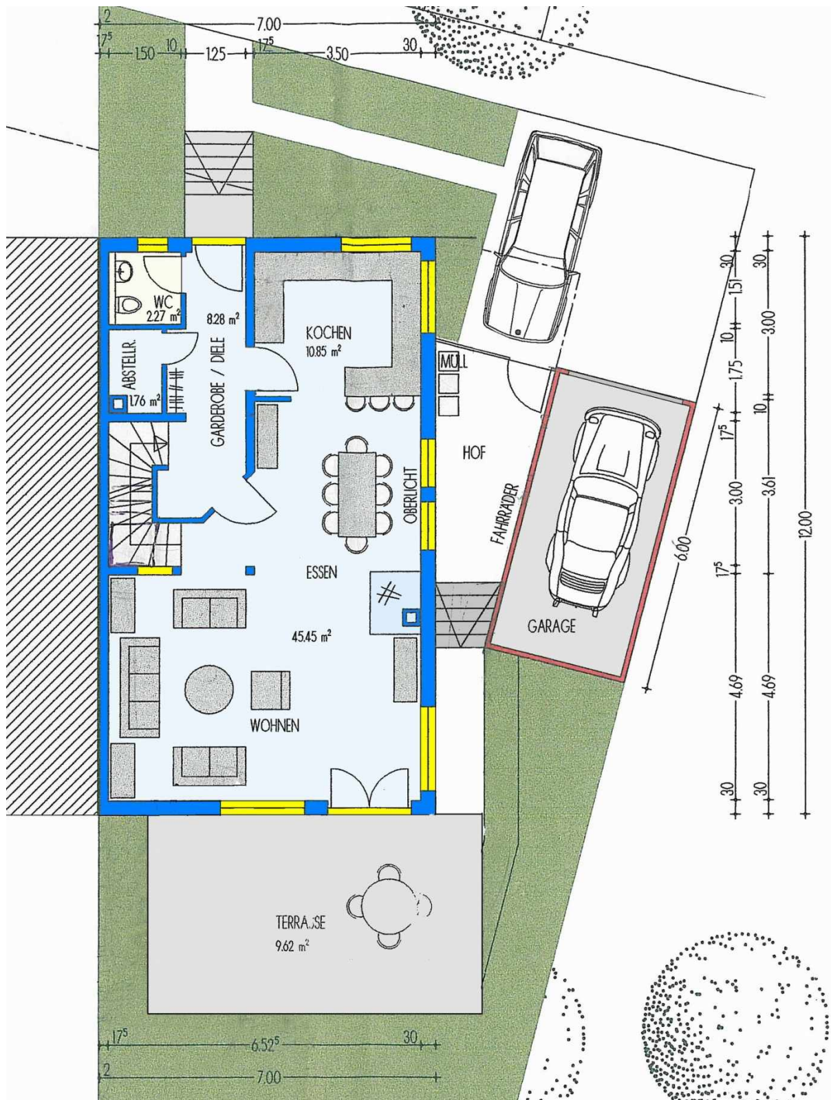
Grundriss Erdgeschoss
